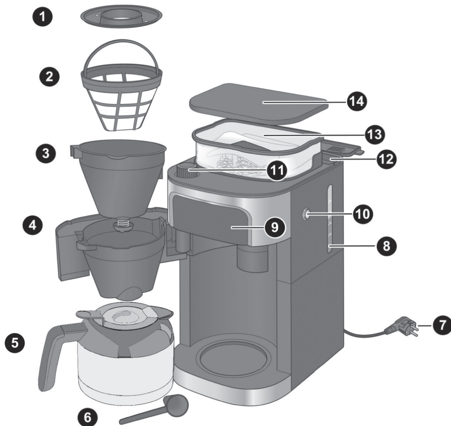
Kuva 1: Laitteen osat
